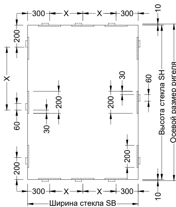
Схема остекления
