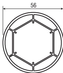
2.1.13 Профиль трубы для эркерных окон арт. 5813
